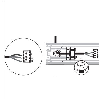
Aansluiting (max. 3x2.5mm 2 )
