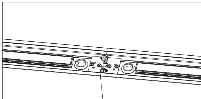
Lijnmontage - Doorvoerbedrading 3x1.5mm 2 / 5x1.5mm 2 DALI
