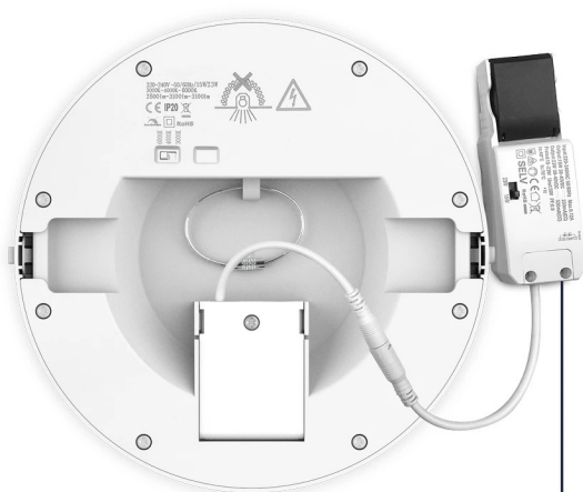
EXTERNE DRIVER Simpele af/aan koppeling
